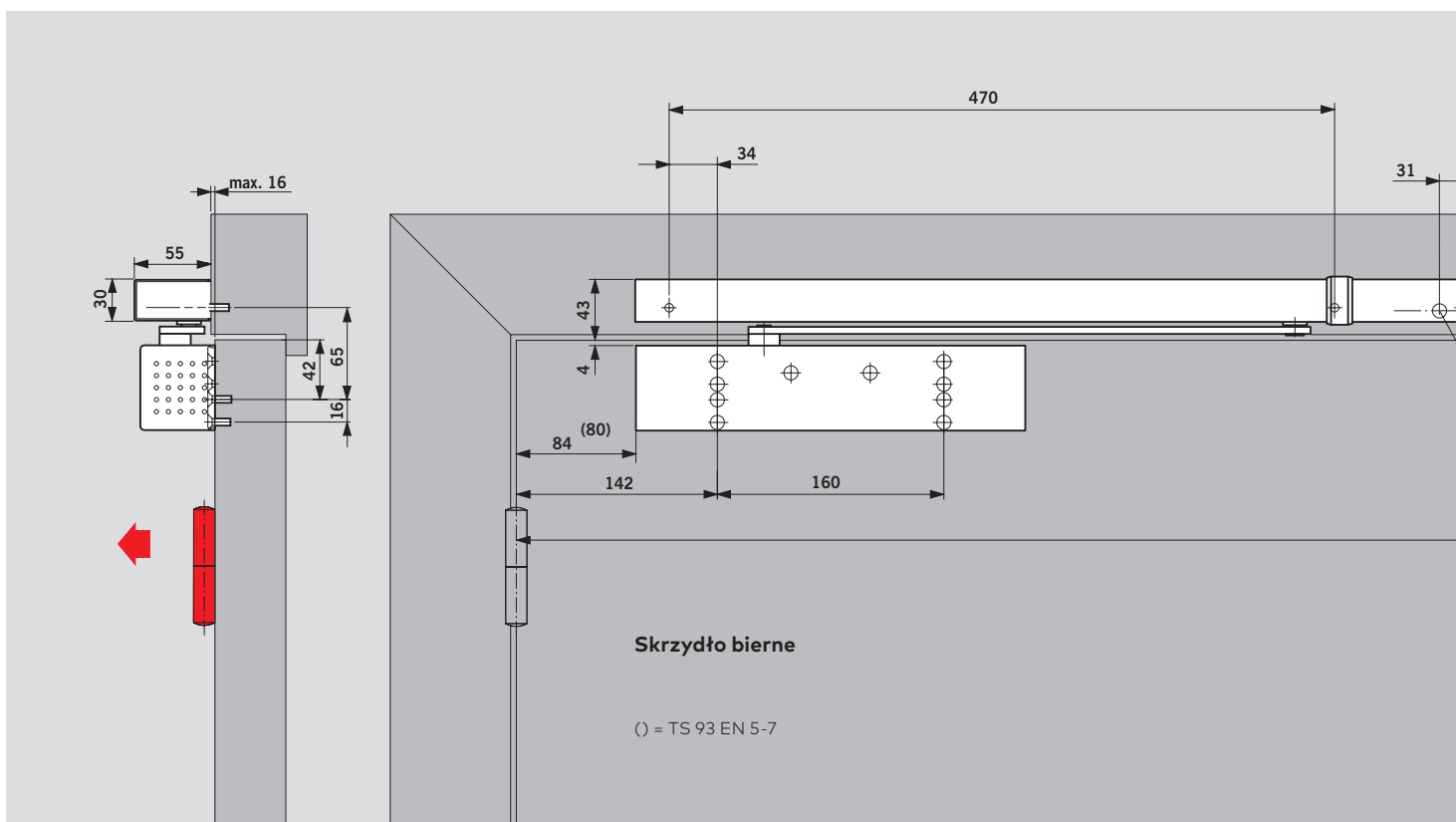
Koordynator ze zintegrowanym czujnikiem dymu (G-SR-EMR)
